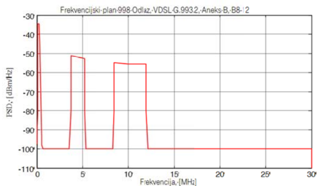
Slika 5.6.3 Frekvenzijski predložak za odlazni smjer prijenosa za VDSL2, frekvenzijski plan 998, B8-12
