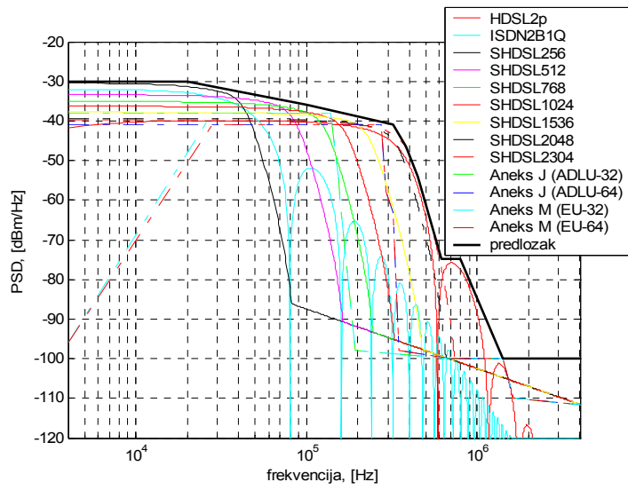
Slika 5.6.1 Frekvenijski predložak za odlazni smjer prijenosa (kratke pretplatničke linije).
