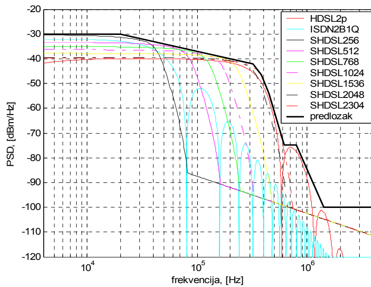
Slika 5.1.1 Frekvenzijski predložak i maske spektralne gustoće snage za simetrične sustave prijenosa.
