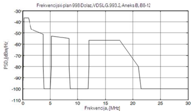
Slika 4.8.4 Maska PSD za VDSL2 frekvenjski plan 998, B8-12 dolaz (crno).
