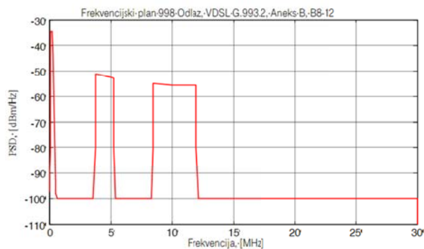
Slika 4.8.5 Maska PSD za VDSL2 frekvenjski plan 998, B8-12 odlaz (crveno)
